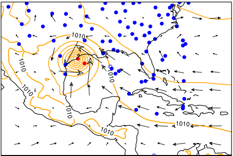
(d) CERA-20C
