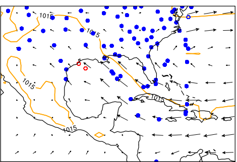
(d) CERA-20C
