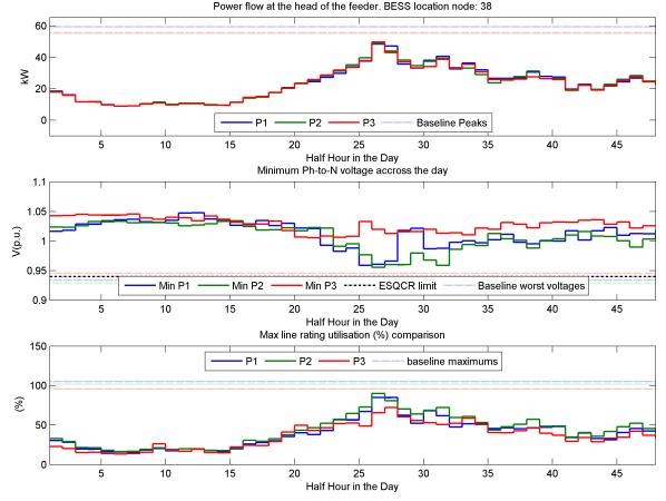
(d) Phase-balancing and storage
