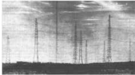
Teilansicht des ersten KW-Antennensterns mit 70-m-Türmen. Ganz links der 70-m-Holzturm mit dem KW-Rundstrahler, Mitte ein 210-m-Mast für LW (1934)
